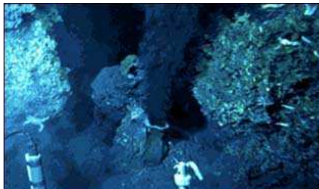
Bild 3: Black Smokers
