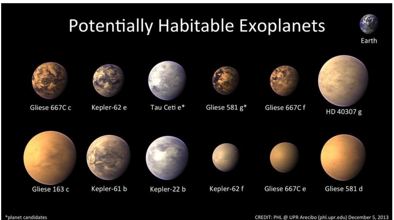
Bild 9: Potentielle Kandidaten von extrasolaren Planeten in einer habitablen Zone um einen Stern
