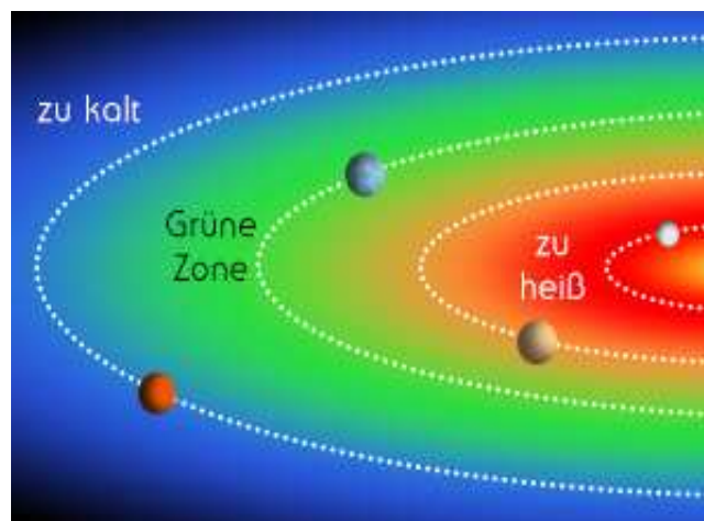
Bild 4: Die habitable Zone um einen Stern
