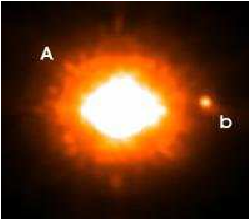
Bild 7: Extrasolarer Planet b um einen Stern A
